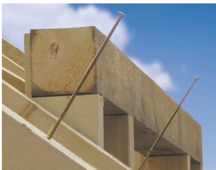
De HECO-TOPIX® als spantgordinganker
